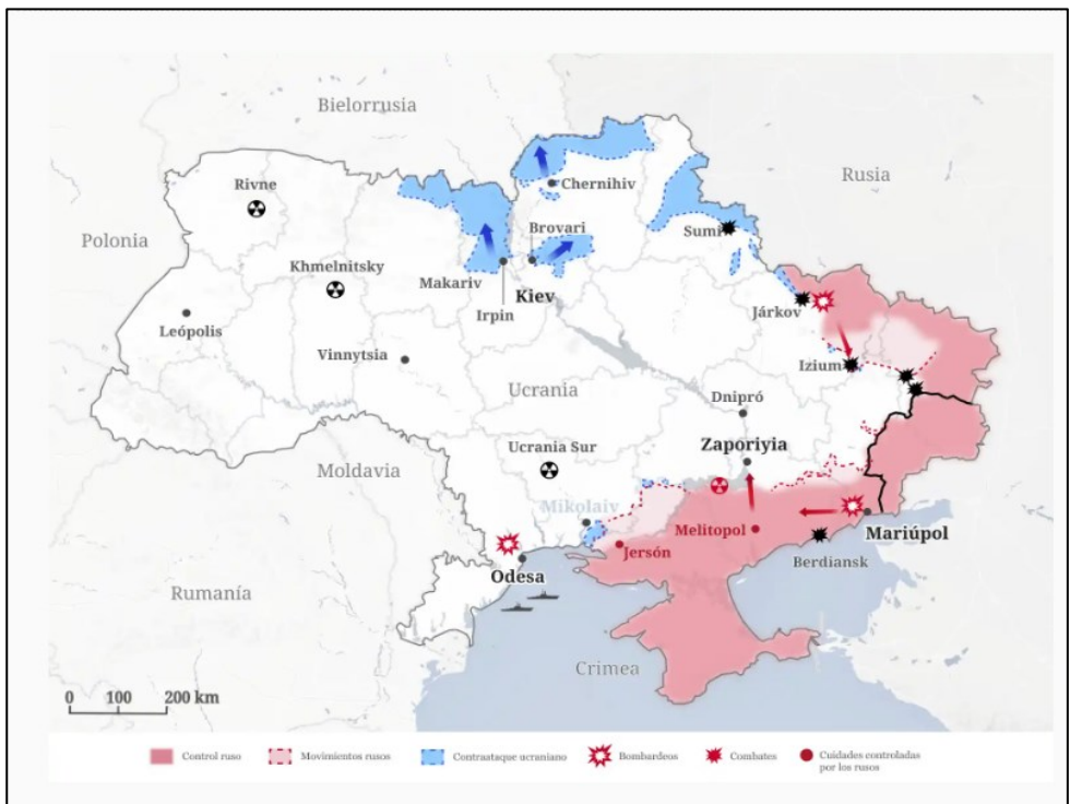
Mapa de la retirada rusa desde Kiev y Chernigov, durante la 1era semana de abril de 2022
